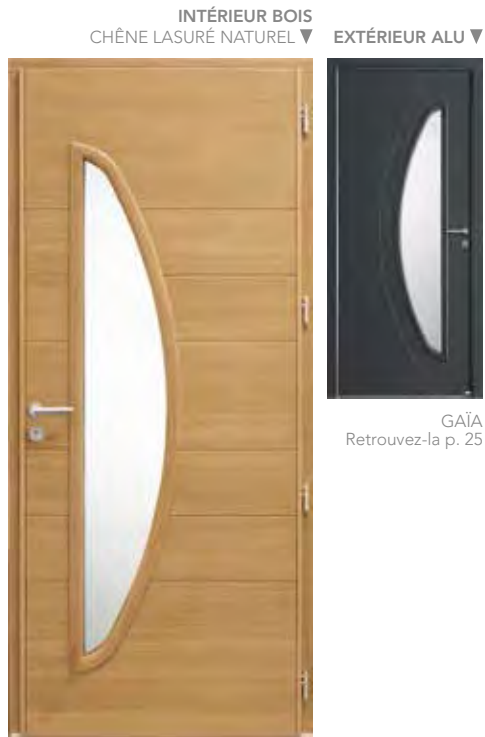
GAÏA Hauteur réalisable : 1900 à 2230 Largeur réalisable : 800 à 1000 Ud=1,3 🔒 🔑 €€€€
