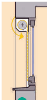
1 Posé sous linteau enroulement extérieur
