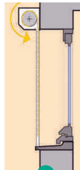
3 Posé devant linteau
