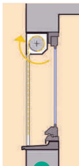
2 Posé sous linteau enroulement intérieur
